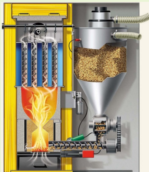
Kocioł na pellet z automatycznym podajnikiem paliwa
