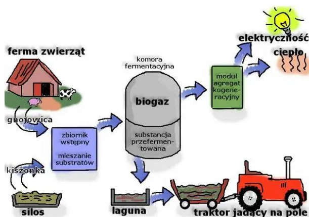
Rys. 20 Schemat produkcji i wykorzystania biogazu
