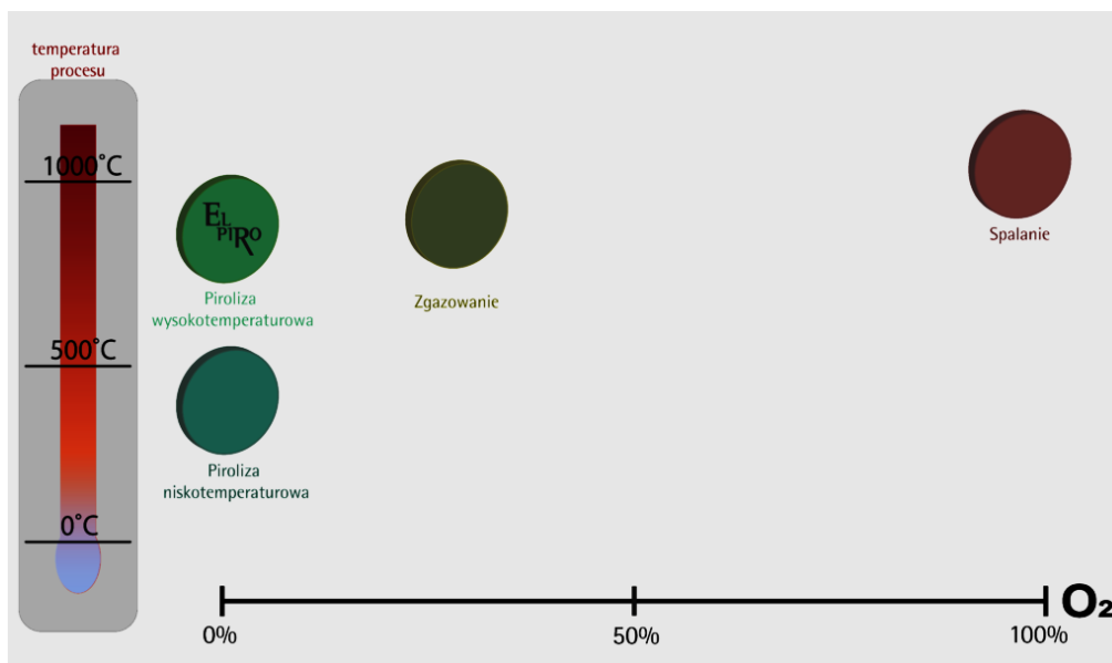
Rys. 19 Porównanie procesów pirolizy, zgazowania oraz spalania
