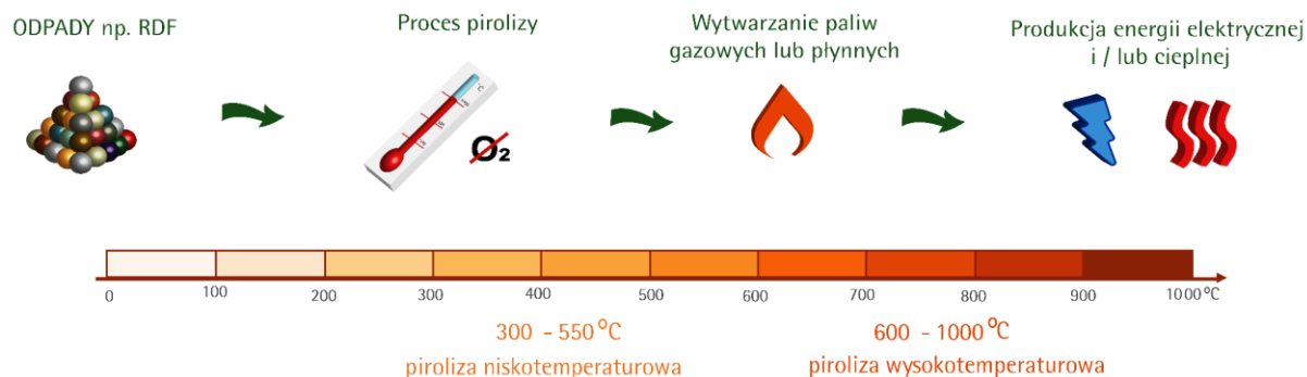
Rys. 14 Przebieg pirolizy
