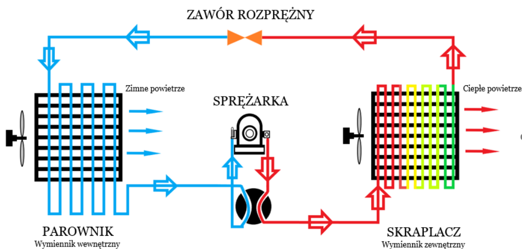
Schemat działania lodówki
