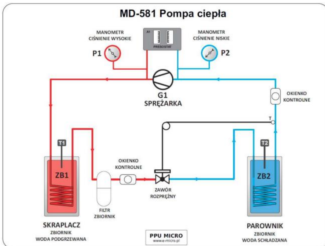
Rys. 1. Schemat stanowiska
